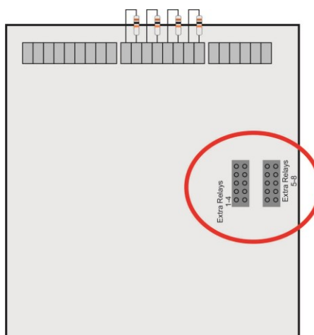
Εικόνα4-13.Σύνδεση επιπλέον ρελέ (for BS-615)
