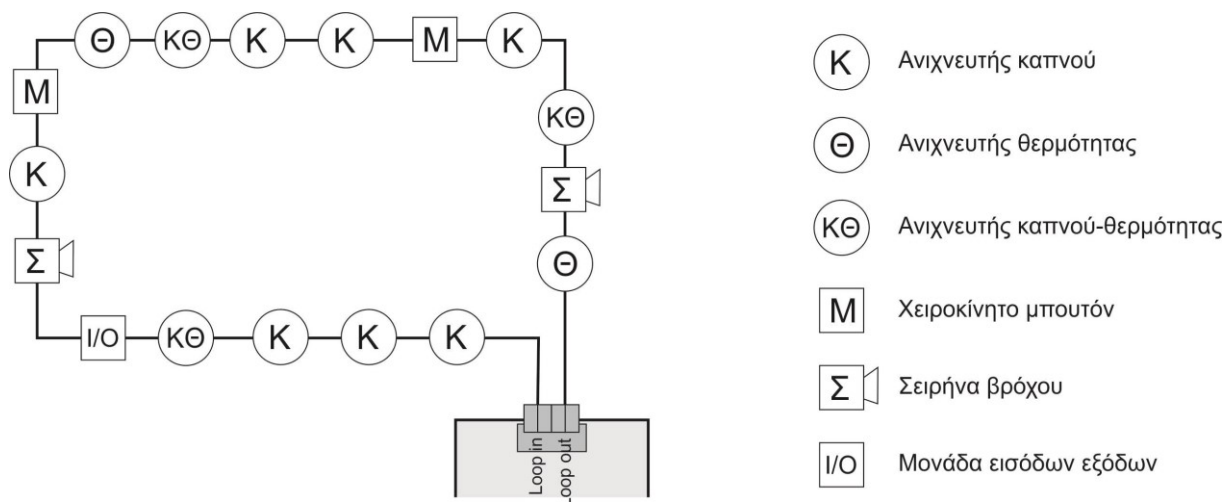
Εικόνα 4-5. Διάγραμμα βρόχου
